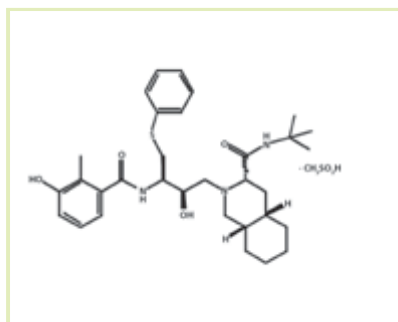
Nelfinavir mesylate.
